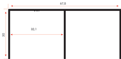
MK 8813 0,455 kg/m
