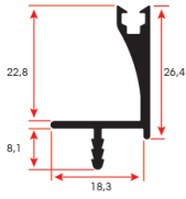
MK 6617 0,425 kg/m
