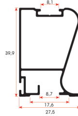
MK 8807 0,515 kg/m
