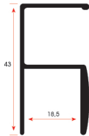
MK 2205 0,315 kg/m
