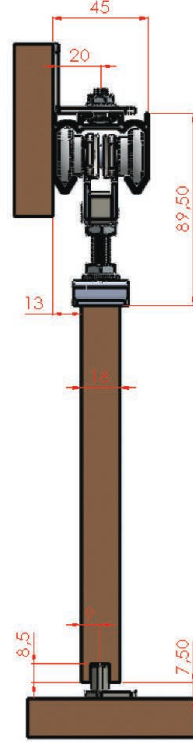
Alt Klavuz Elemanı Bottom Guide Component
