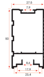
MK 8810 0,220 kg/m
