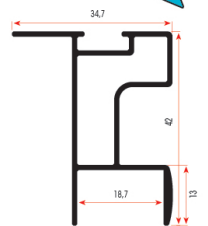
MK 2242 0,475 kg/m
