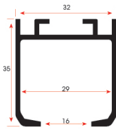
MK 3306 0,520 kg/m
