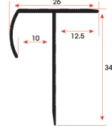
MK 1116 0,190 kg/m
