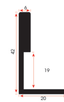
MK 2208 0,630 kg/m
