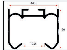
Üst Ray Top Rail
