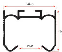
MK 3307 0,620 kg/m
