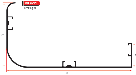
Kapı Kasası Bükümlü Köşe
