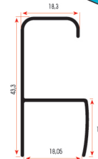
MK 2243 0,275 kg/m
