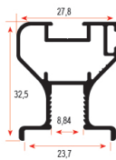
MK 8802 0,400 kg/m
