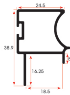
MK 2206 0,410 kg/m
