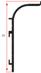
MK 6616 0,290 kg/m
