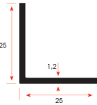
MK 1104 0,160 kg/m
