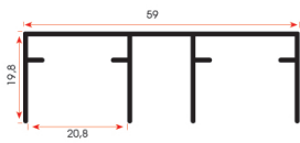
MK 3309 0,410 kg/m
