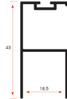
MK 2208 0,630 kg/m
