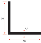
MK 1109 0,105 kg/m
