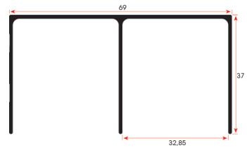
MK 8814 0,550 kg/m
