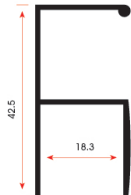
MK 2206 0,410 kg/m
