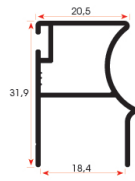
MK 2207 0,320 kg/m
