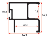
MK 2205 0,315 kg/m
