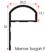
MK 6604 0,250 kg/m
