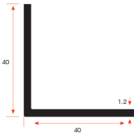
MK 1110 0,110 kg/m
