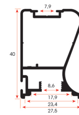
MK 8812 0,360 kg/m
