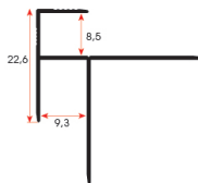
MK 1115 0,213 kg/m
