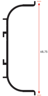
MK 6617 0,425 kg/m
